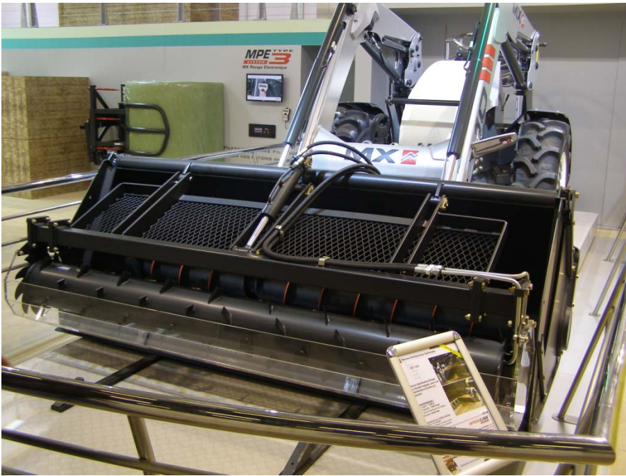
Skopa försedd med rotor som river ner foder från ett foderlager. Också från MX.
